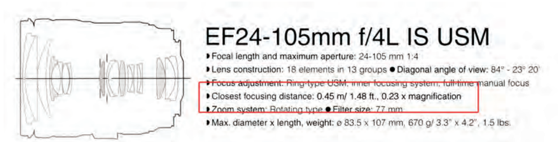
Specificaties van een lens met onder andere de kortste scherpstelafstand en de afbeeldingsmaatstaf (vergrotingsfactor).
